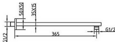
Braço de ducha mural cuadrado. Square wall shower arm.
