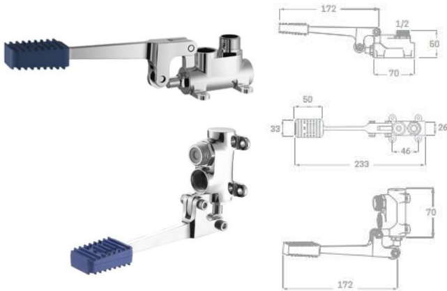
Flujómetro pedal 1 agua. Instalación pared o suelo. Pedal flushometer 1 water. Wall or floor installation.
