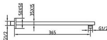
Braço de ducha mural cuadrado. Square wall shower arm.
