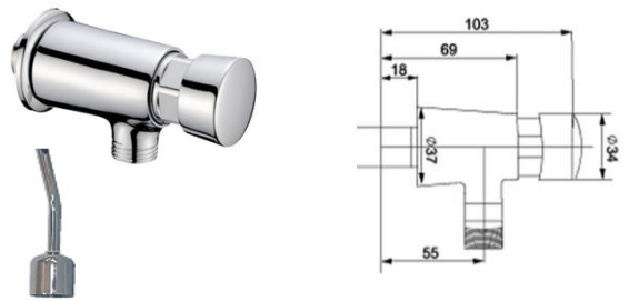
Flujómetro para urinario. Duración del caudal 8-12 segundos.
