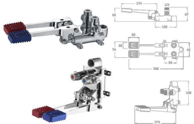
Flujómetro pedal 2 aguas. Instalación pared o suelo. Pedal flushometer 2 waters. Wall or floor installation.
